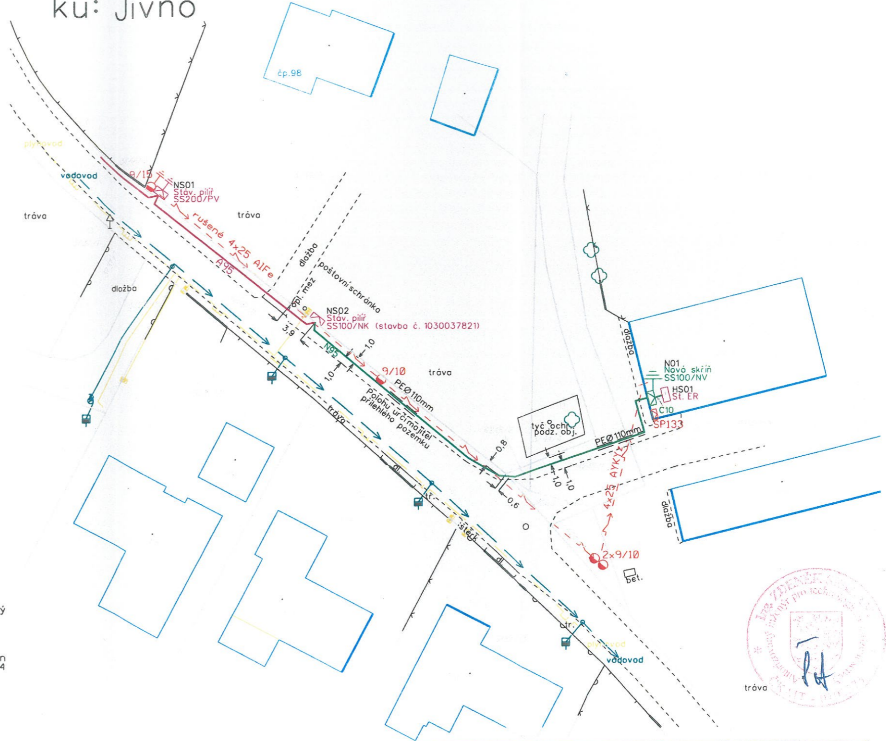
ULOŽENÍ FeZn 30/4
