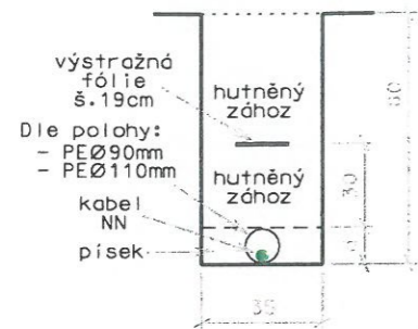
PŘEKOP NEZP. VJEZDU A POJEZDOVÉ PLOCHY V NEZP. CESTĚ
